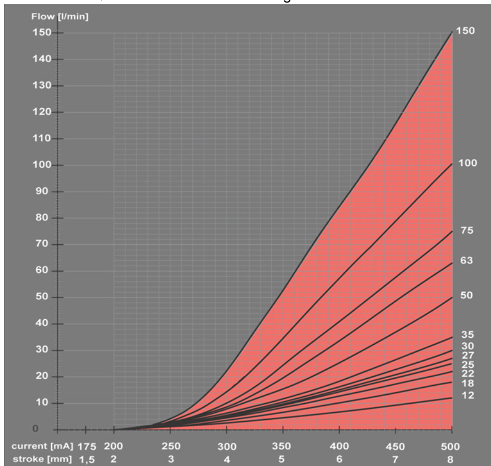
Diagram: Proportionellt flöde från Olsbergs lastkännande och tryckkompen-serade ventil Q300 med mekanisk återföring av sliden.
